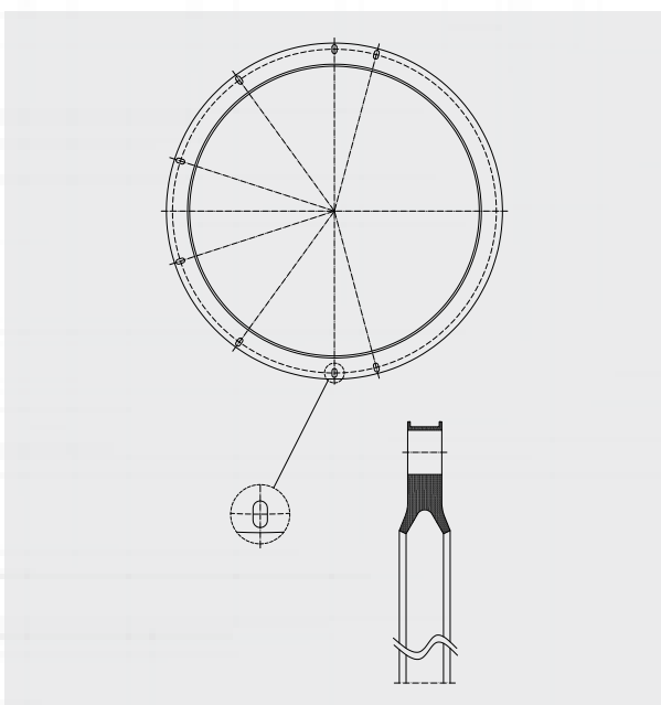
Anel de Vedação 850x986 seção Y para Filtro Hiperbarico 40622
